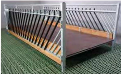
Futtertischgang 3,00m-Elemente
